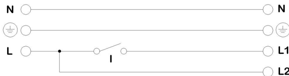
fig. 2 – collegamenti elettrici
