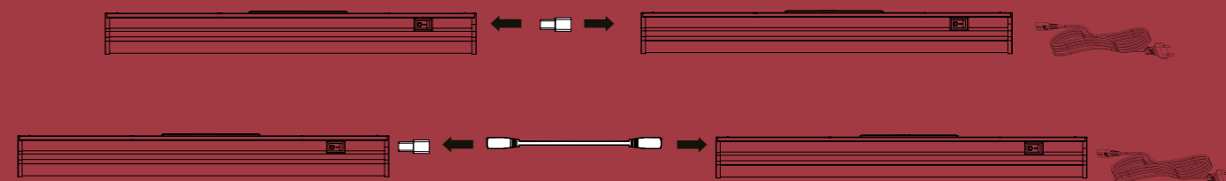
Collegamento di Miniled CCT con connettori in dotazione
