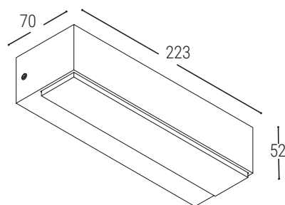
Tratto CCT mono emissione
