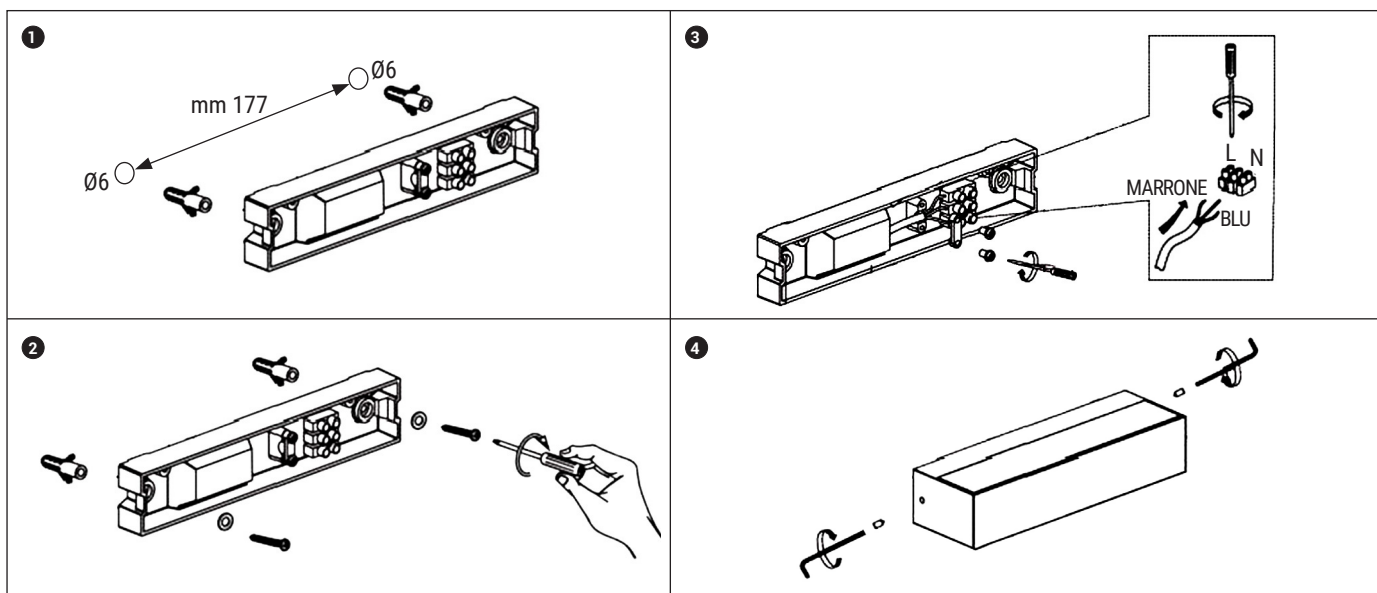
Tratto 2 CCT bi emissione
