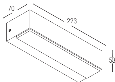
Tratto 2 CCT bi emissione
